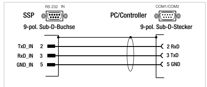
Bild 1 Verbindungskabel für serielle Schnittstelle
